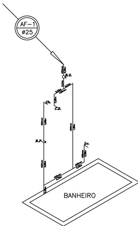
ISOMÉTRICO-1
