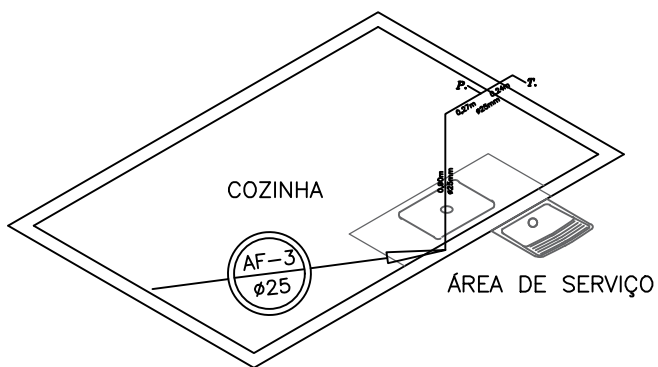
ISOMÉTRICO-2
