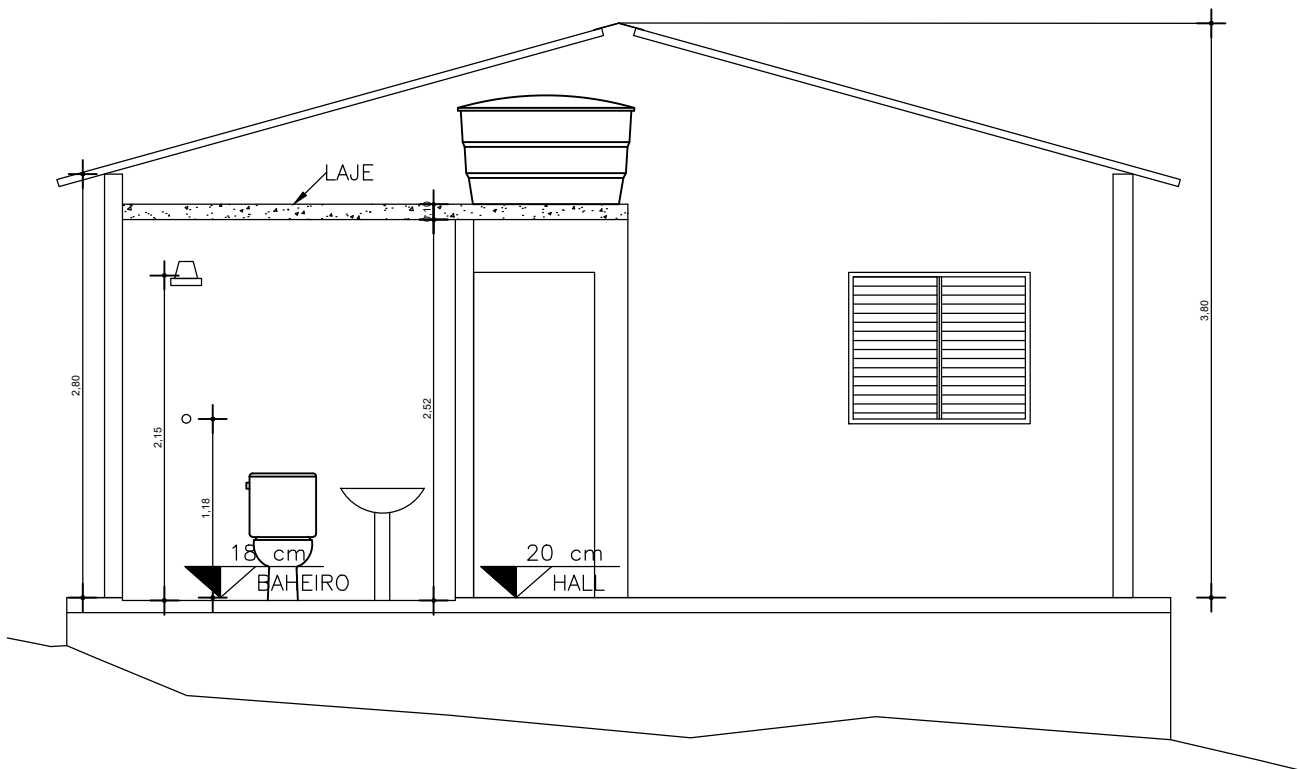
CORTE A-A
