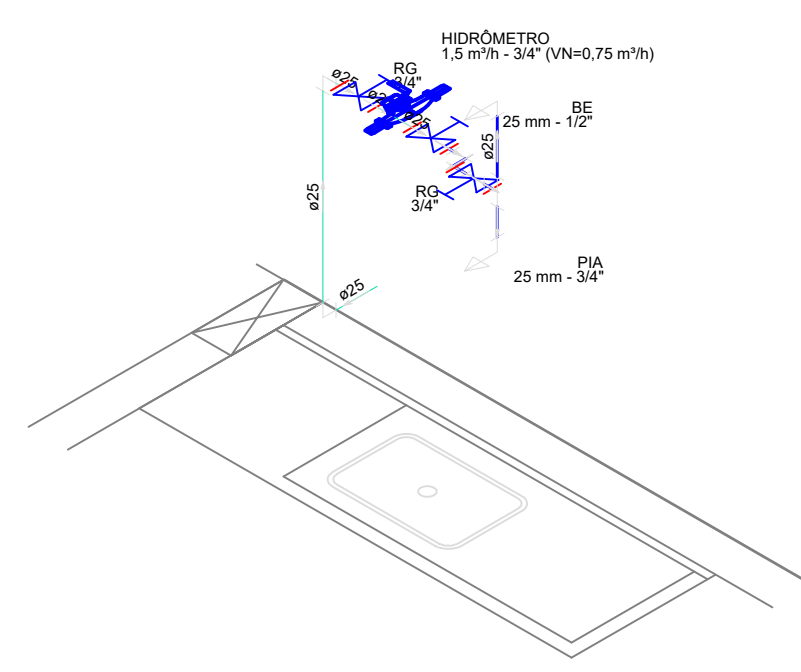
DETALHE QUIOSQUES 1A14-1 Escala 1:25
