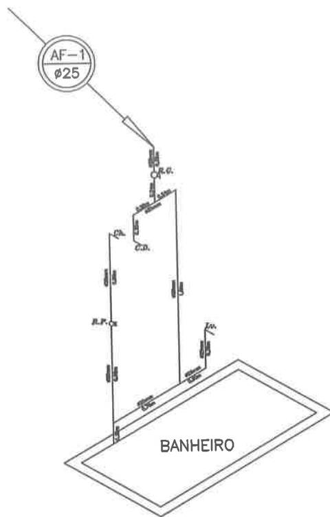
ISOMÉTRICO-1
