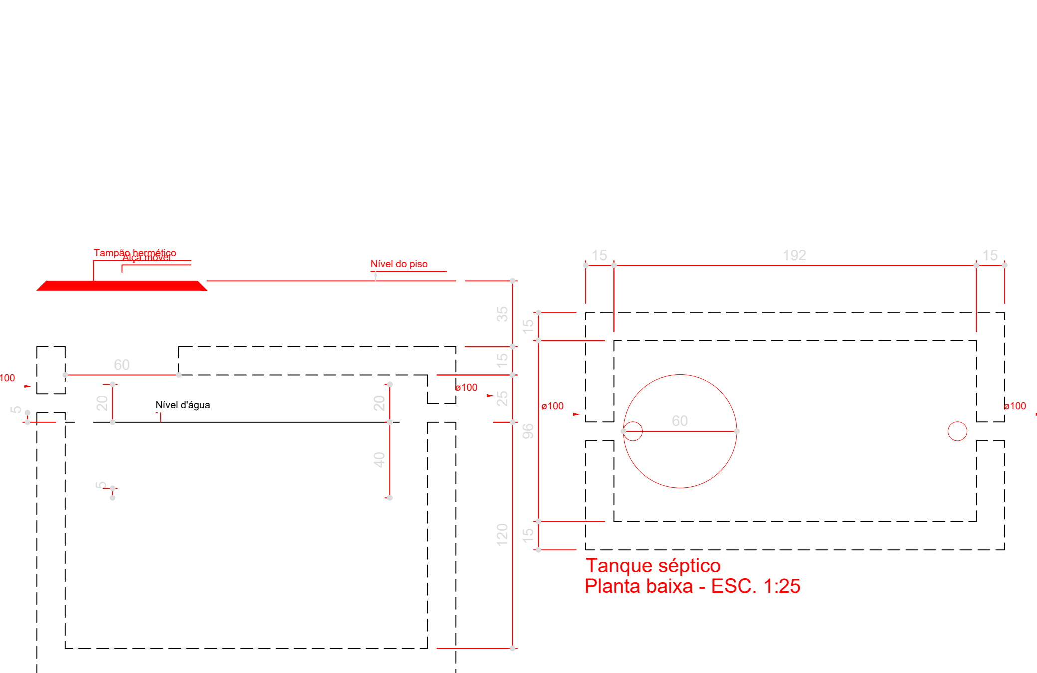
Tanque séptico CORTE 1 - ESC. 1:25
