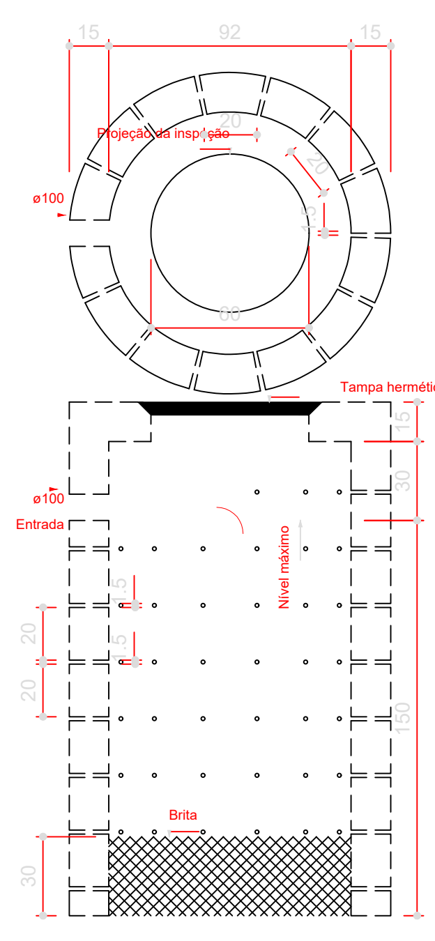
Sumidouro CORTE 1 - ESC. 1:25
