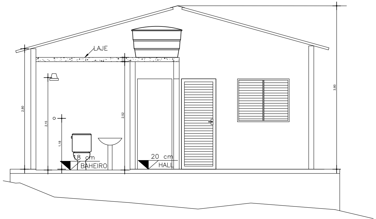
CORTE A-A
