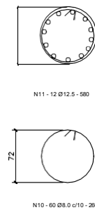
TUBULÕES (X4) PROFUNDIDADE 6 m
