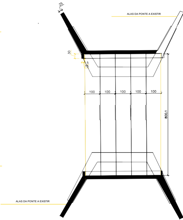
REFORÇO PEGÕES EXISTENTES Esc.: 1:100
