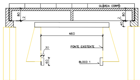
REFORÇO PEGÕES EXISTENTES Esc.: 1:100
