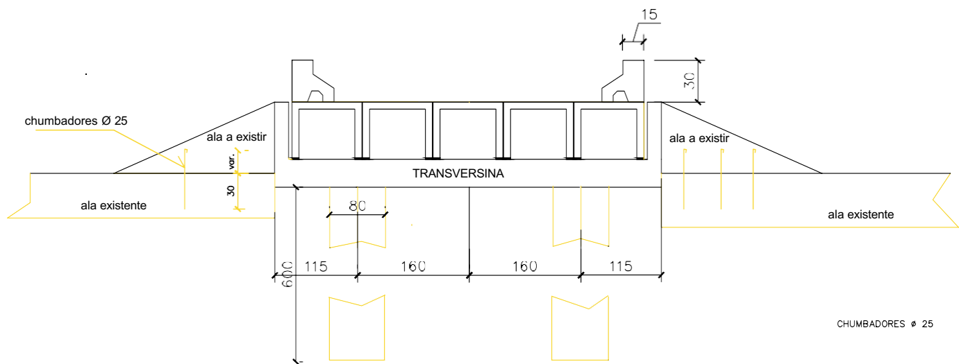
DEIALHE DOS PEGÕES
