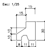
DETALHE GUARDA CORPO
