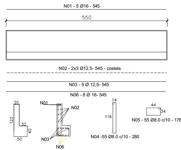
TRANSVERSINA CORTINA (X2) Esc.: 1/50
