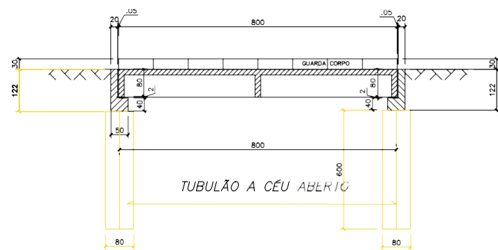
PERFIL LONGITUDINAL Esc.: 1:100
