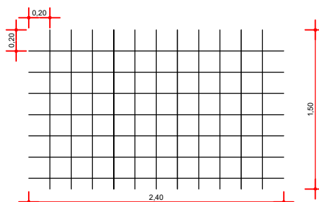
MALHA PARA LAJE 20X20 - Ø6.3mm (1/4") S/Esc.
